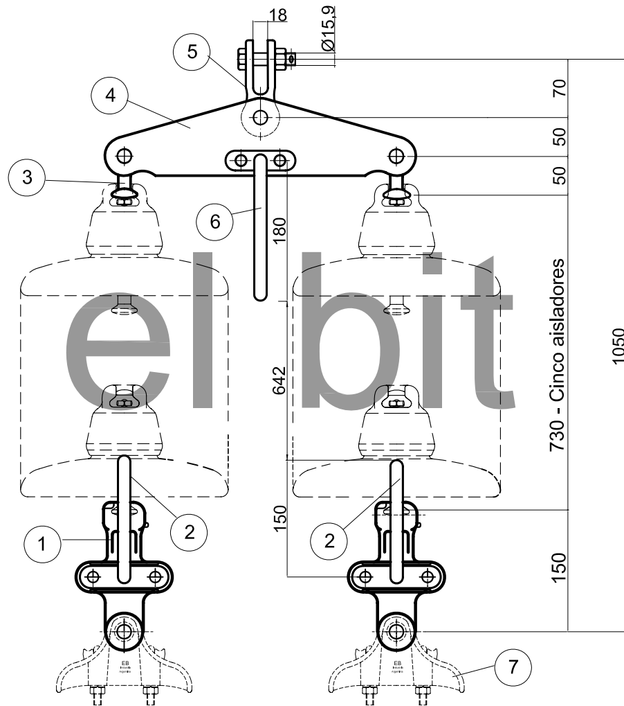
BADAJO y ORBITA: Dimensiones según Norma UTE NO-DIS-MA-4009
